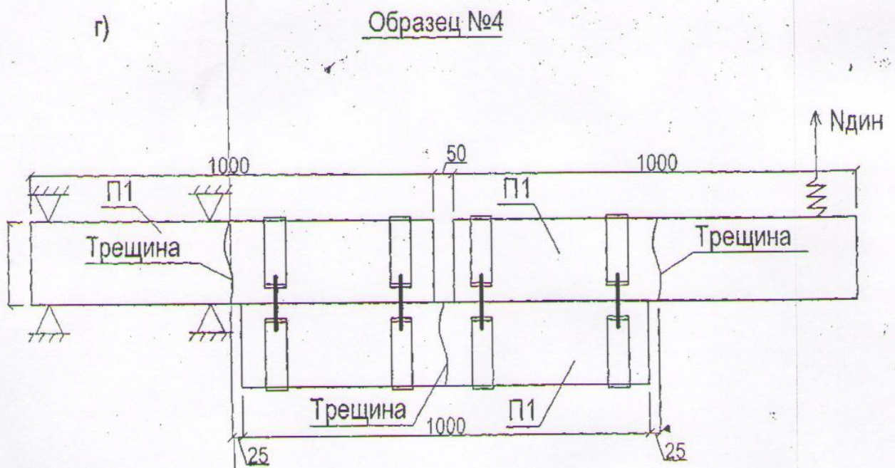
Рис. 3.2. Схемы испытаний блоков со стеклопластиковой арматурой.
