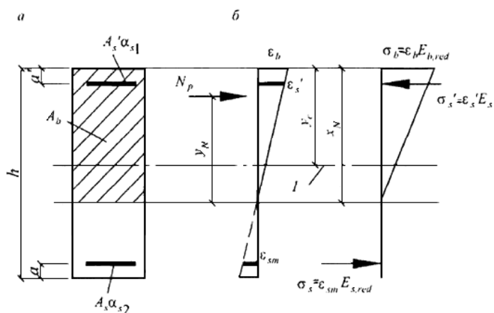
Рисунок 9.3 - Приведенное поперечное сечение и схема напряженно-деформированного состояния изгибаемого предварительно напряженного элемента с трещинами при его расчете по деформациям
