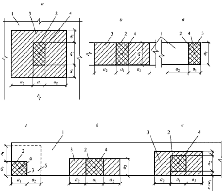
а - вдали от краев элемента; б - по всей ширине элемента; в - у края (торца) элемента по всей его ширине; г - на углу элемента; д - у одного края элемента; е - вблизи одного края элемента.
