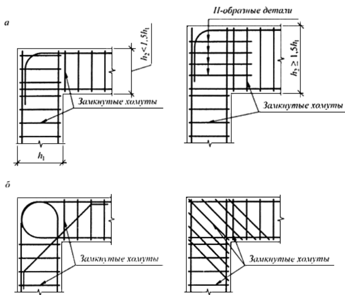
Рисунок 10.2 - Узлы сопряжения балок с колоннами
