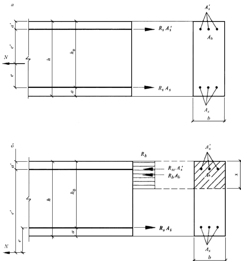
Рисунок 8.4 - Схема усилий и эпюра напряжений в сечении, нормальном к продольной оси внецентренно растянутого железобетонного элемента, при расчете его по прочности при применении продольной силы
