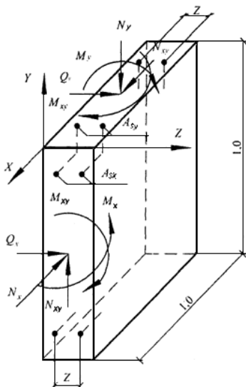
Рисунок 8.16 - Схема усилий, действующих на выделенный плоский элемент единичной ширины стены
